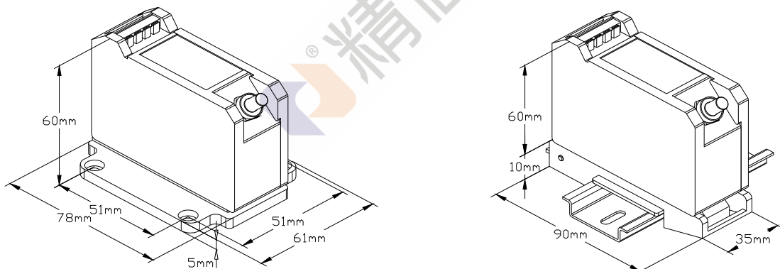
图1-7 前置器
