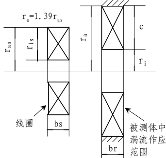
图1-8 被测体中电涡流效应范围
