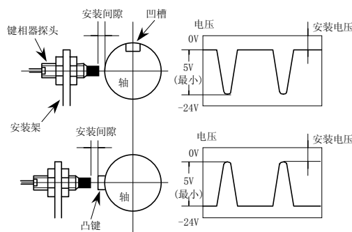
图 2-5 键相器测量
