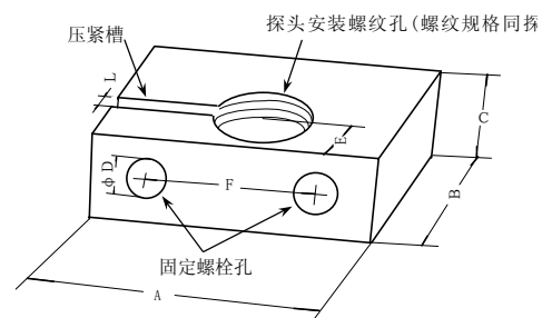
图2-10 夹块支架
