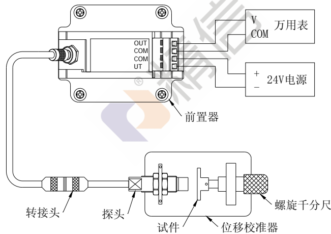
图 3-1 校准安装示意图
