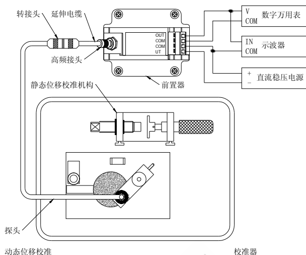
图 B-8 用校准仪进行动态特性试验
