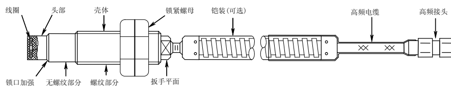
图1-5 探头典型结构
