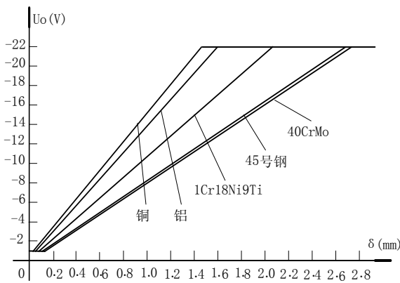
图1-9 典型材料传感器输出特性曲线
