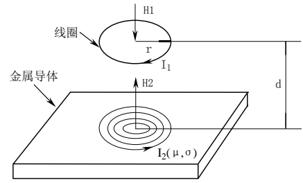
图 1-2 电涡流作用原理图
