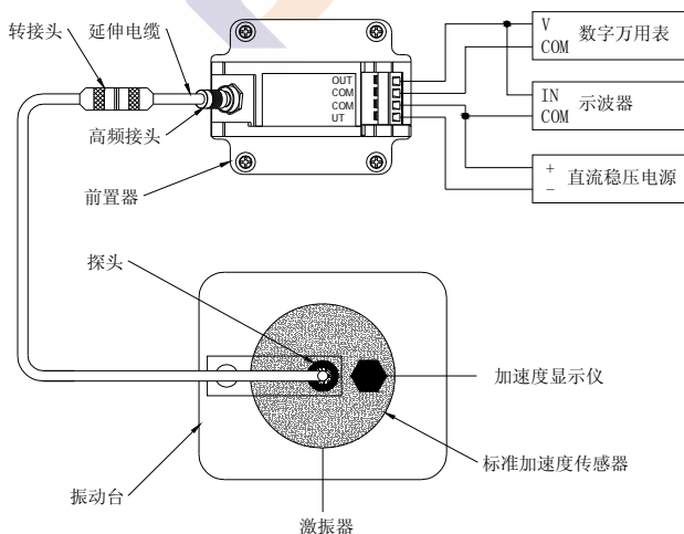
图 B-9 用振动台进行动态特性试验
