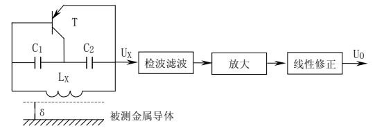
图 1-3 传感器原理框图
