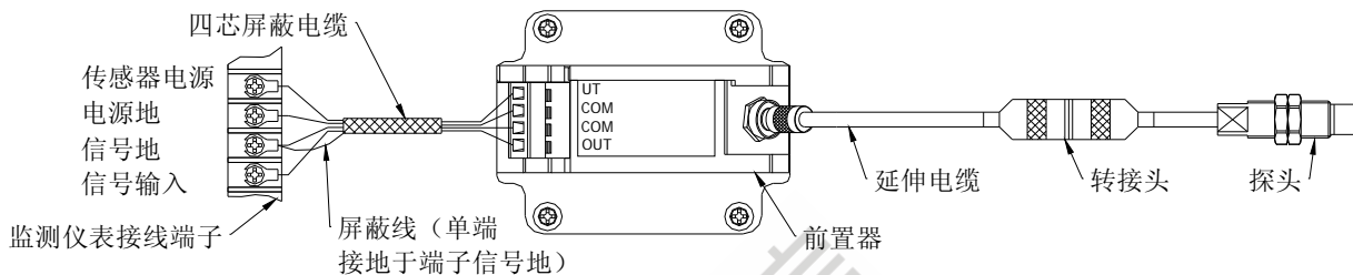
图 2-19 系统连接示意图
